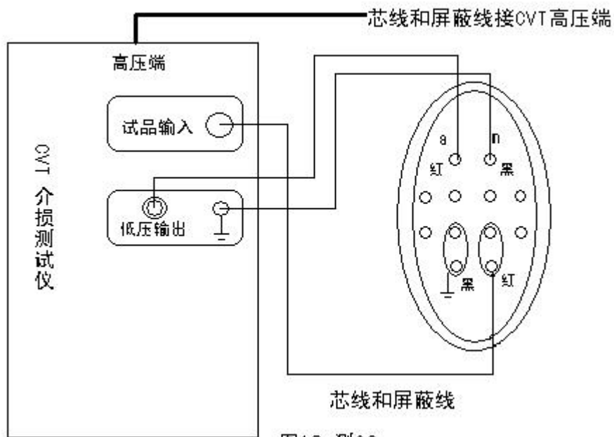
图13 测C2
