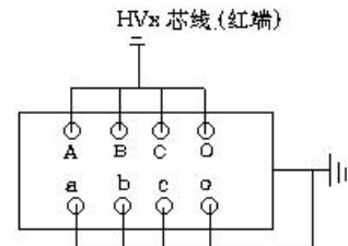
图 12 变压器接法
