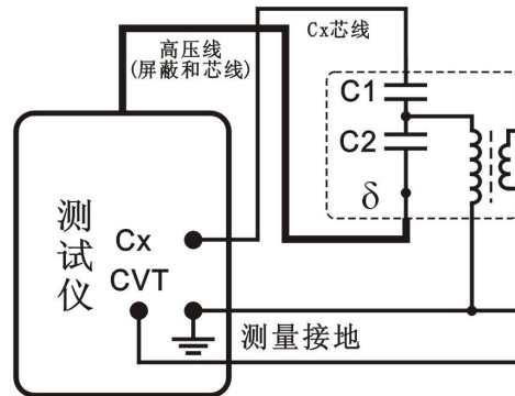
CVT (测量C1) 接线示意图
