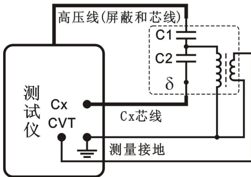
CVT (测量C2) 接线示意图
