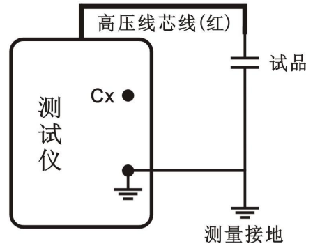
反接线示意图
