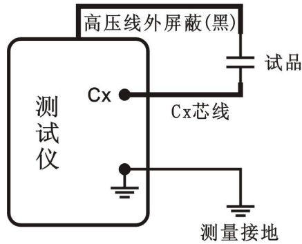
正接线示意图
